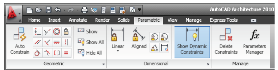
Figure 1: Parametric palette
